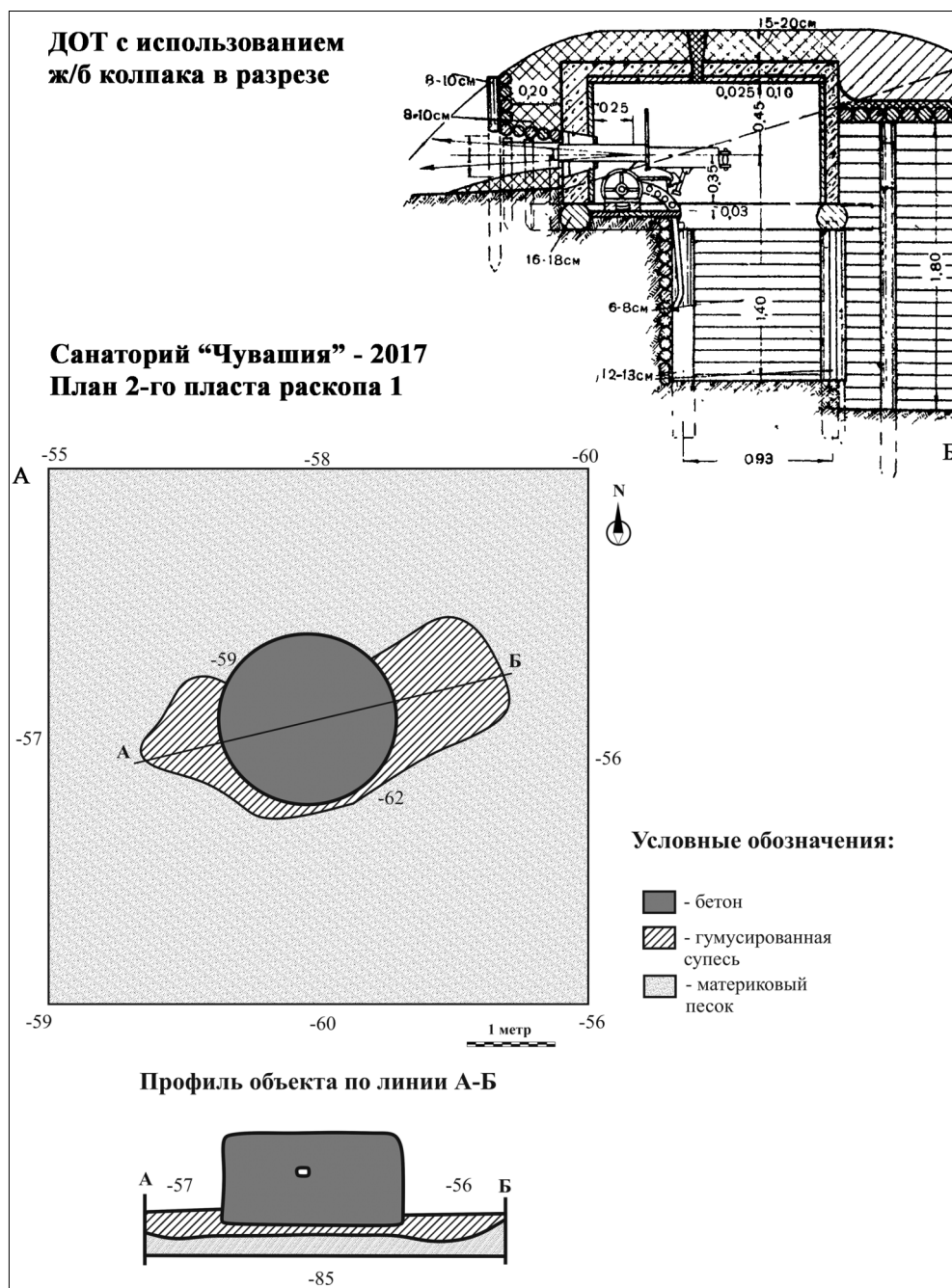
Рис. 4. План 2-го пласта в раскопе № 1 2017 г. и профиль объекта (ж/б колпака) по линии А-Б (А). Долговременная огневая точка (ДОТ) с использованием железобетонного колпака в разрезе // Наставление для инженерных войск. Полевая фортификация (ПФ-43). Ч. 2. Фортификационные сооружения. М., 1946. С. 30, 33—34 (Б)
