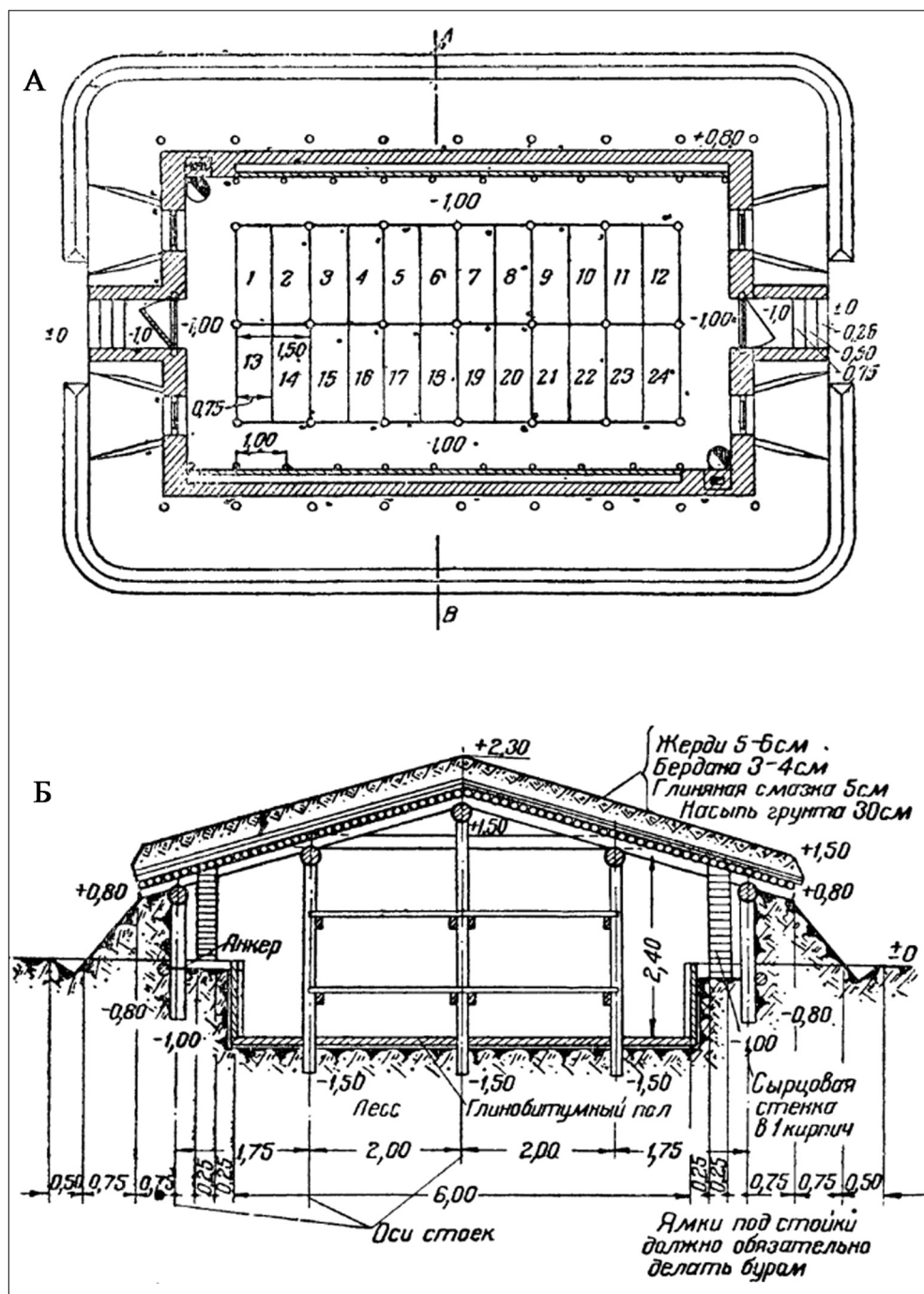
Рис. 7. План (А) и разрез (Б) полууглубленной землянки // Полевые необоронительные постройки. Наставления для войск Красной Армии. М.; Л., 1941. Рис. 111—112
