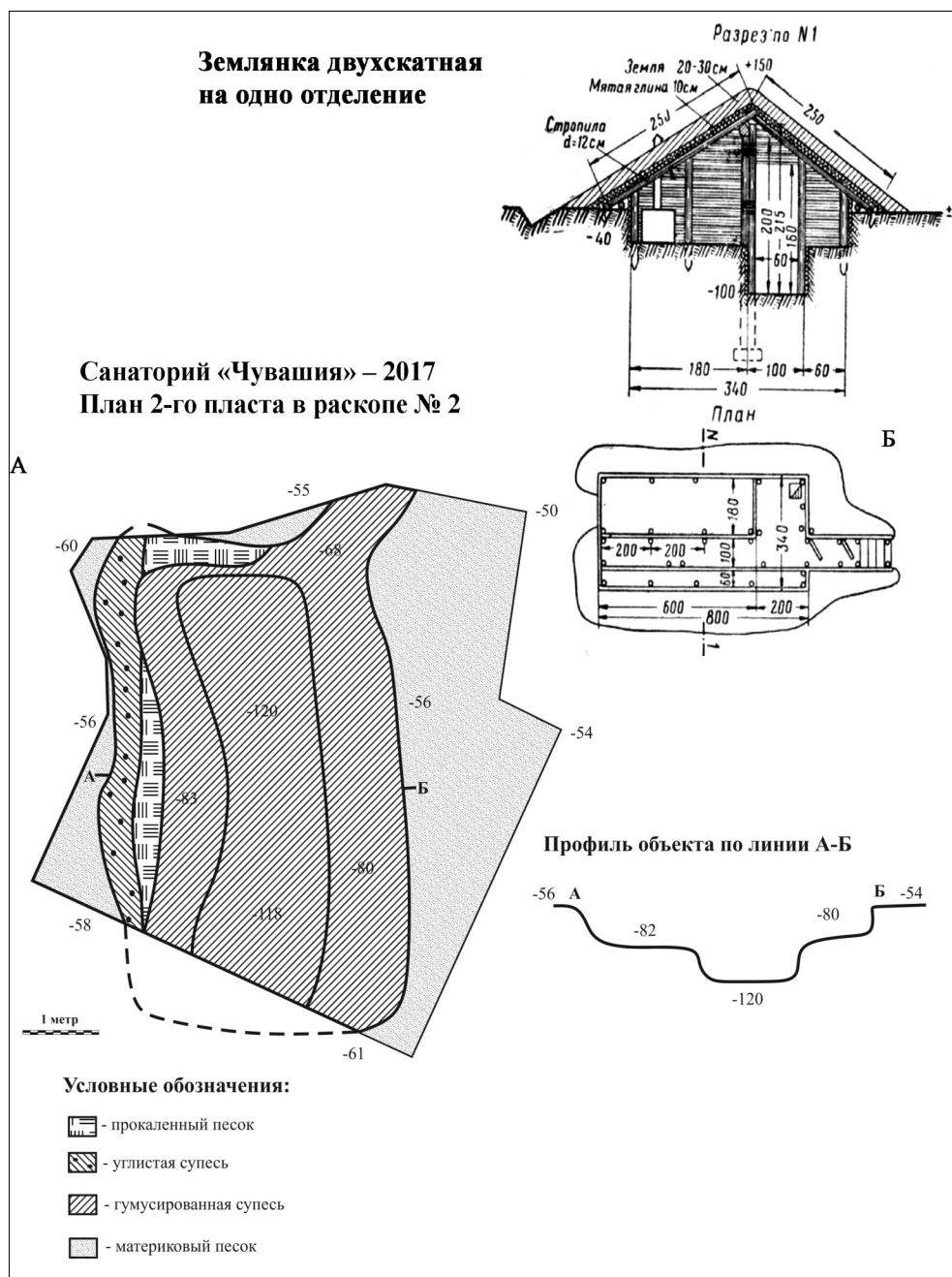
Рис. 6. План 2-го пласта в раскопе № 2 2017 г. и профиль объекта (землянки по линии А-Б (А). Землянка двухскатная на одно отделение // Полевые необоронительные постройки. Наставления для войск Красной Армии. М.; Л., 1941 (Б)
